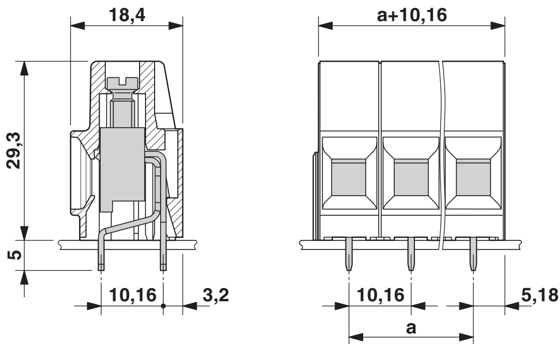
Rysunek wymiarowy
