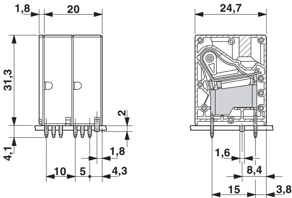
Rysunek wymiarowy
