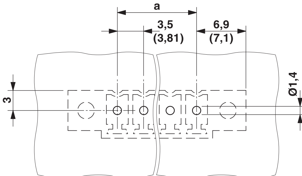
Otworowanie/geometria płytek lutowicznych
