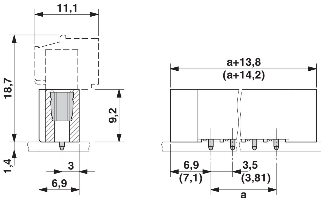
Rysunek wymiarowy
