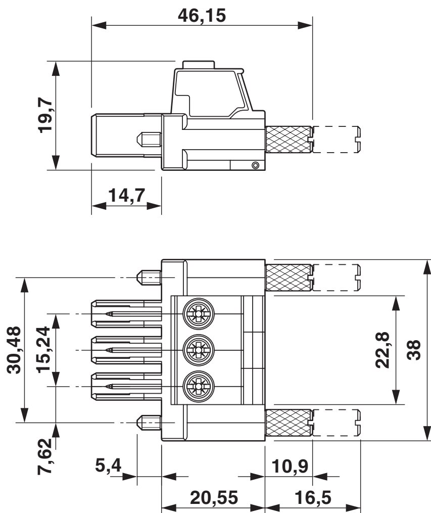
Rysunek wymiarowy
