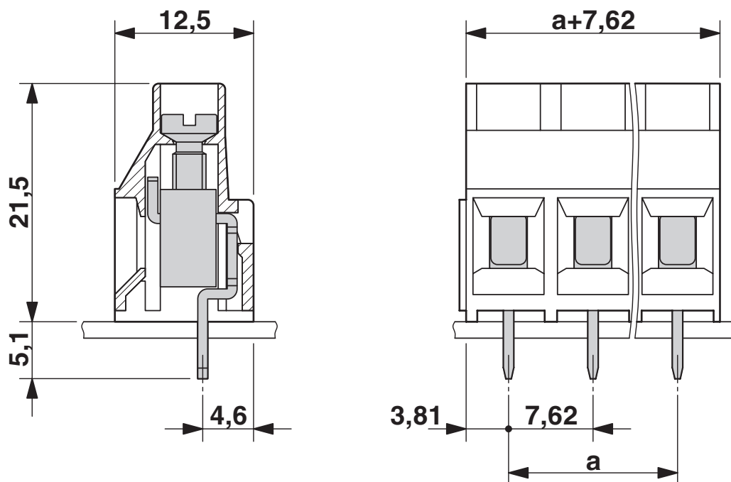
Rysunek wymiarowy
