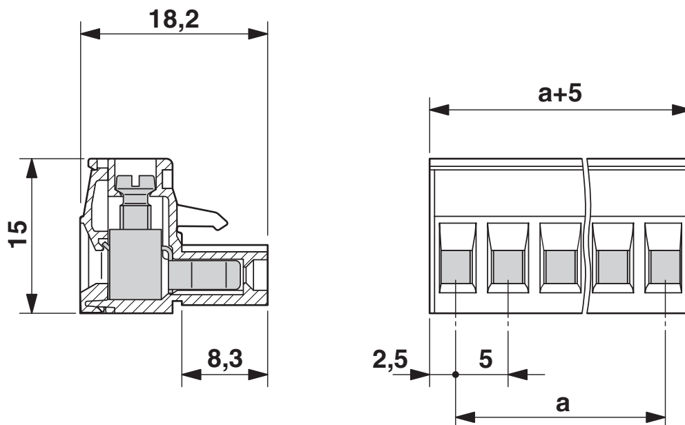
Rysunek wymiarowy
