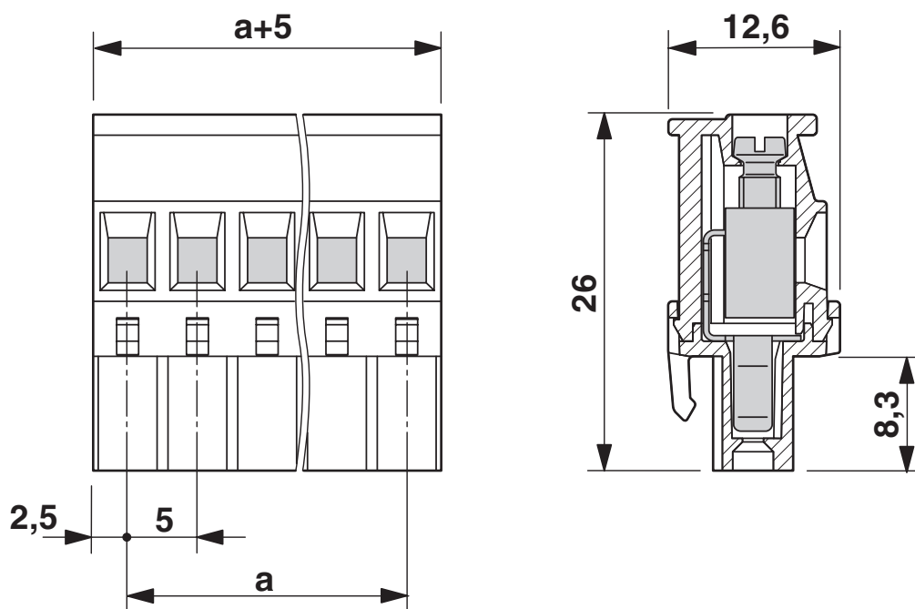
Rysunek wymiarowy
