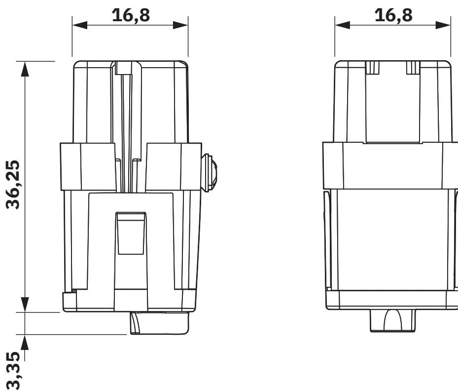
Rysunek wymiarowy
