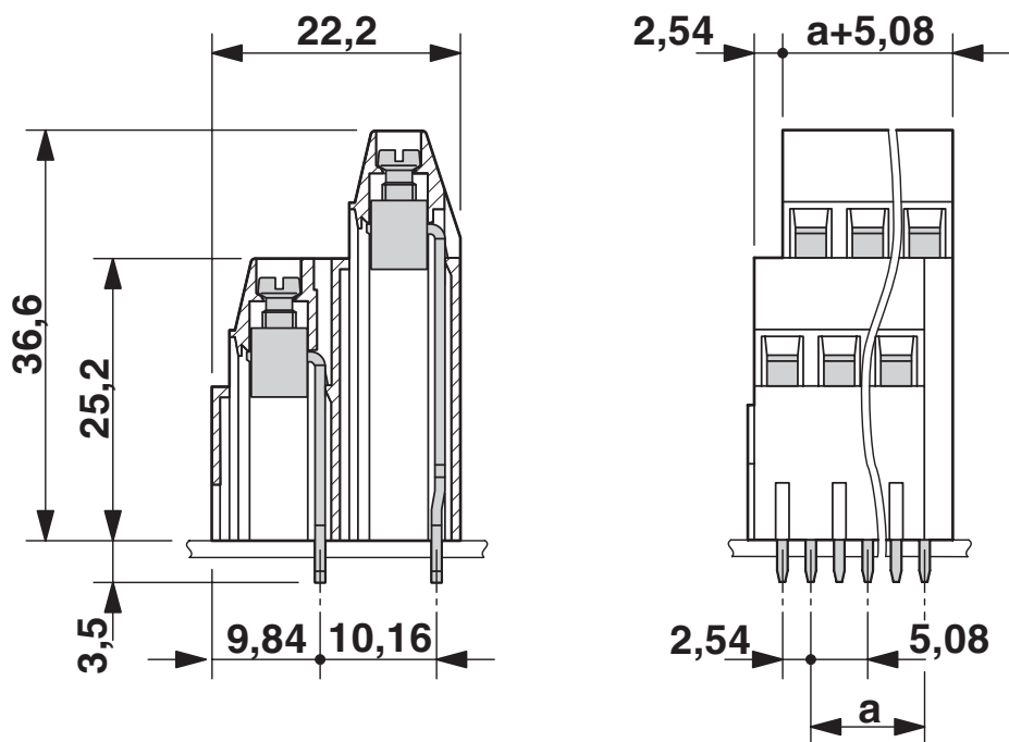
Rysunek wymiarowy
