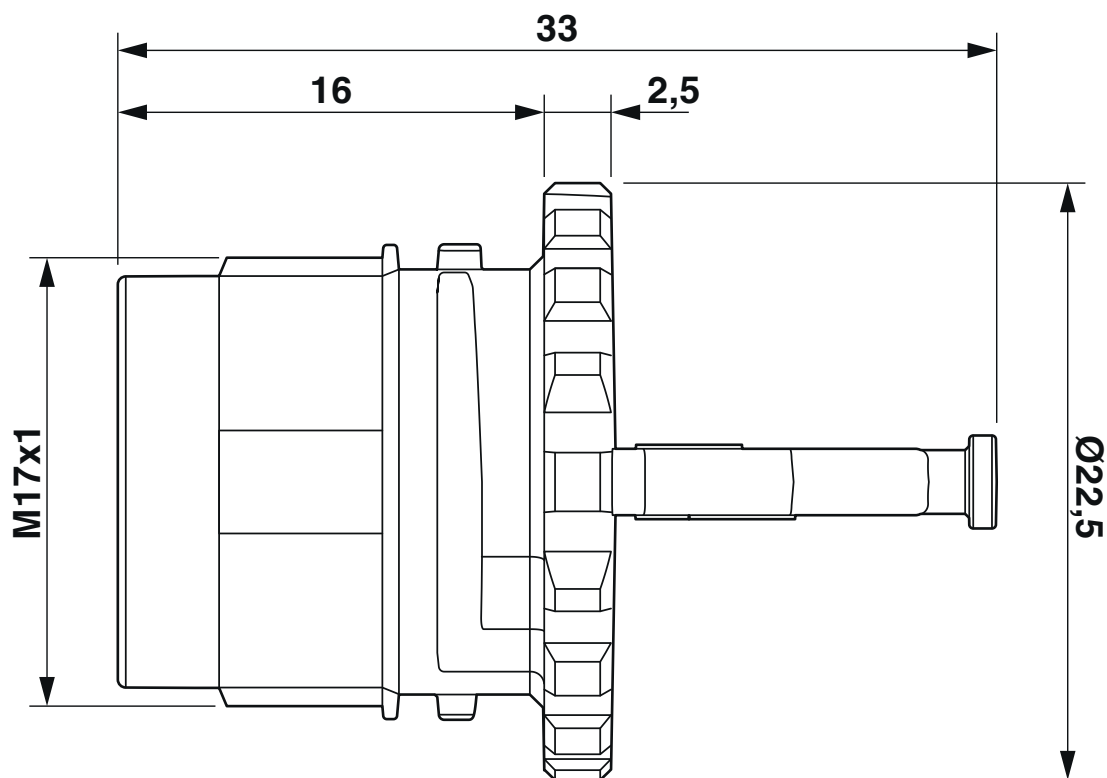
Rysunek wymiarowy
