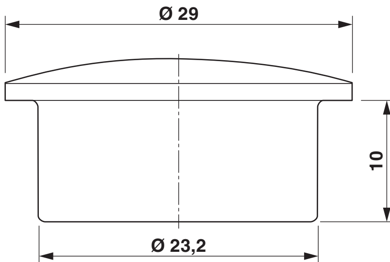
Rysunek wymiarowy
