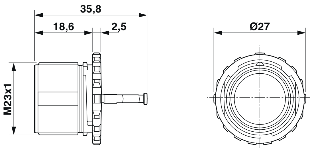
Rysunek wymiarowy
