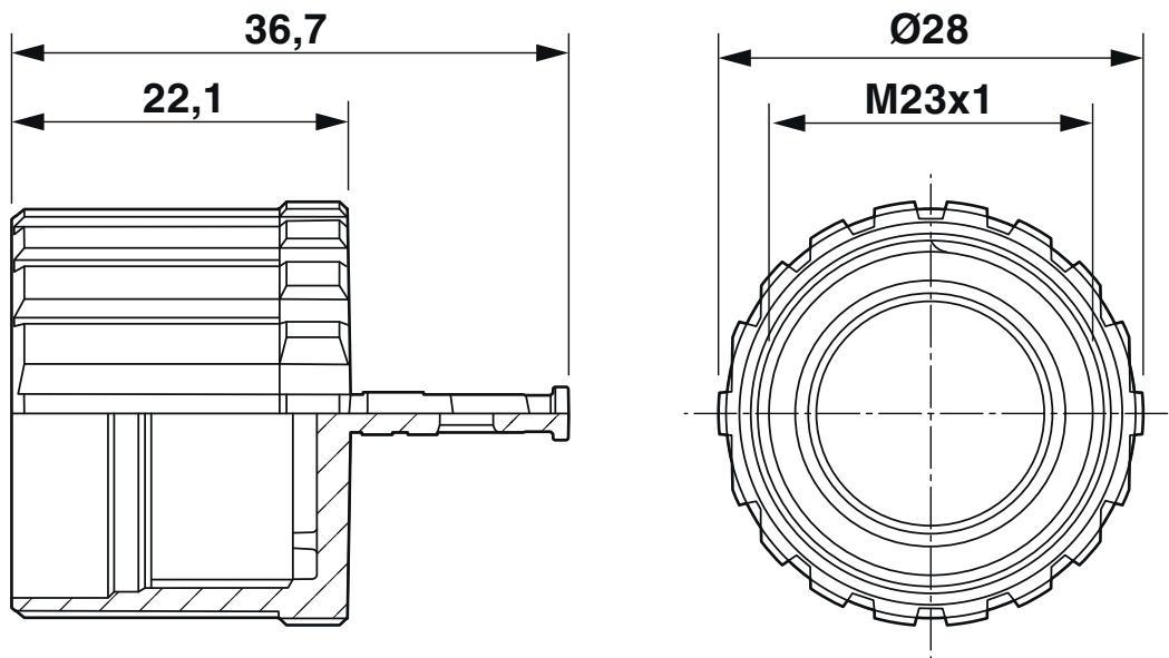
Rysunek wymiarowy
