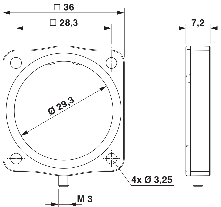
Rysunek wymiarowy
