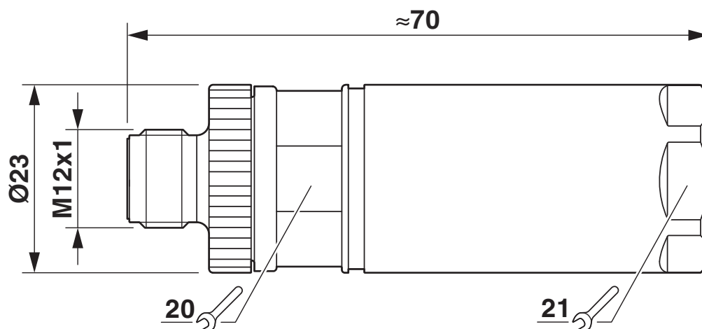
Rysunek wymiarowy
