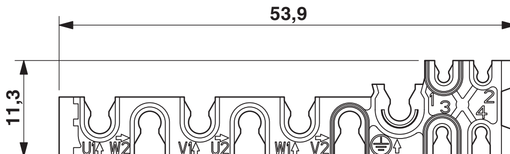
Rysunek wymiarowy
