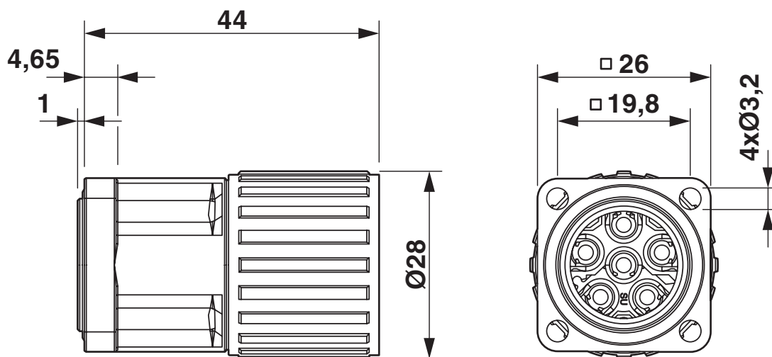
Rysunek wymiarowy
