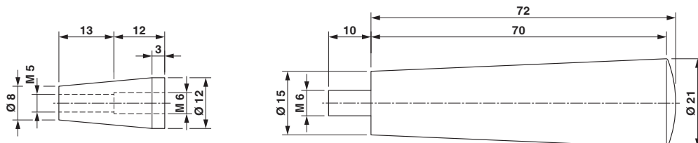
Rysunek wymiarowy
