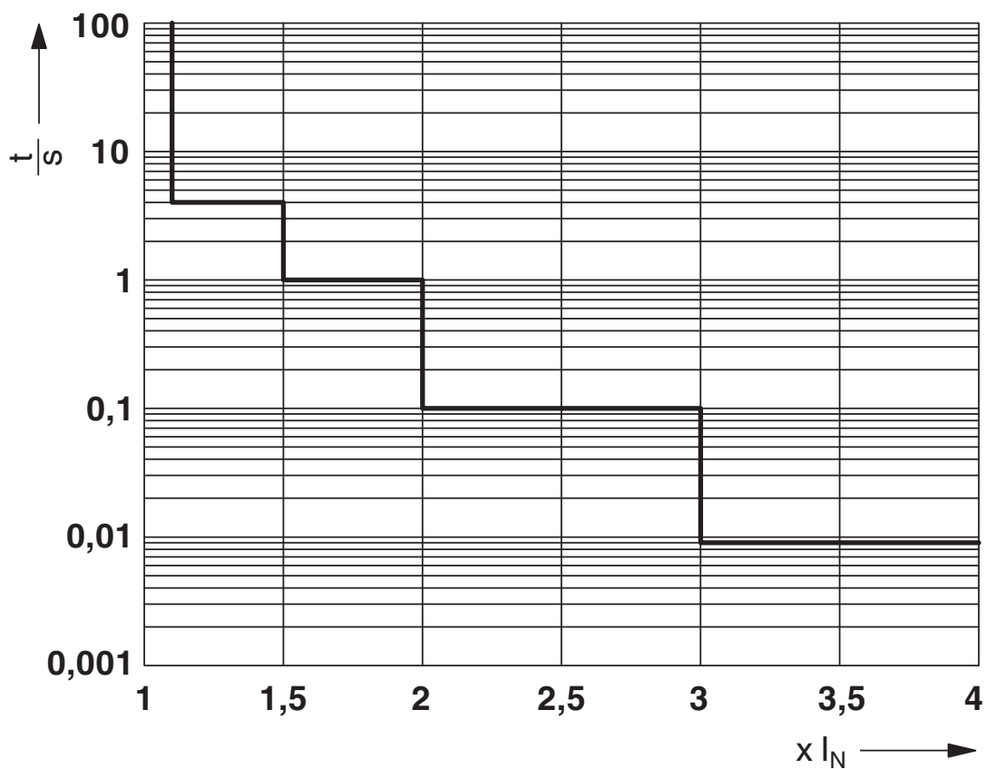
Charakterystyka wyzwalania
