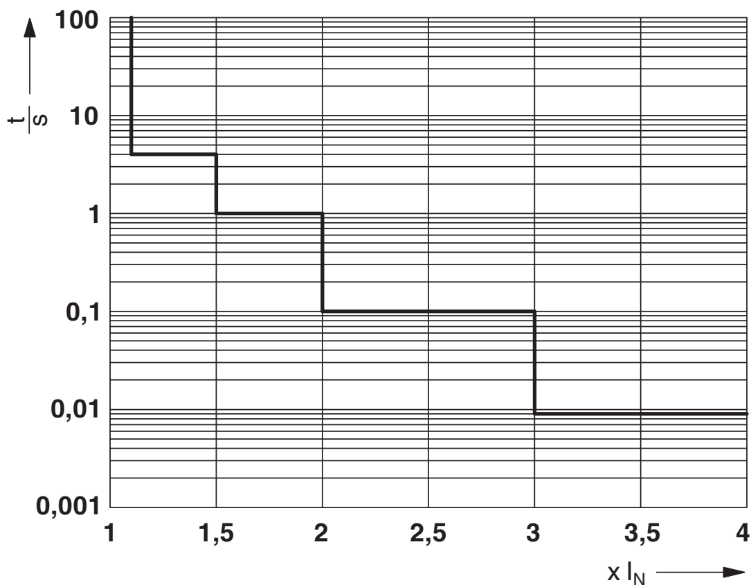
Charakterystyka wyzwalania
