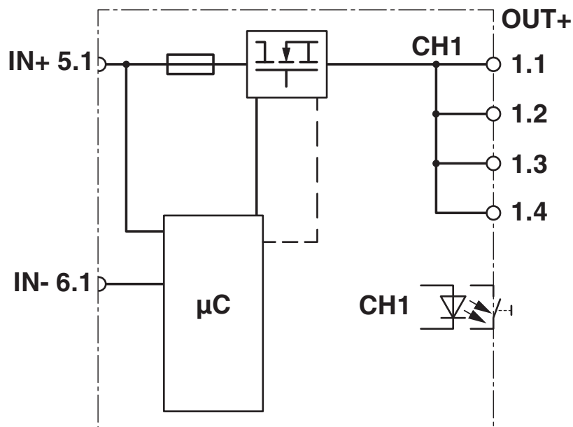
Schemat blokowy
