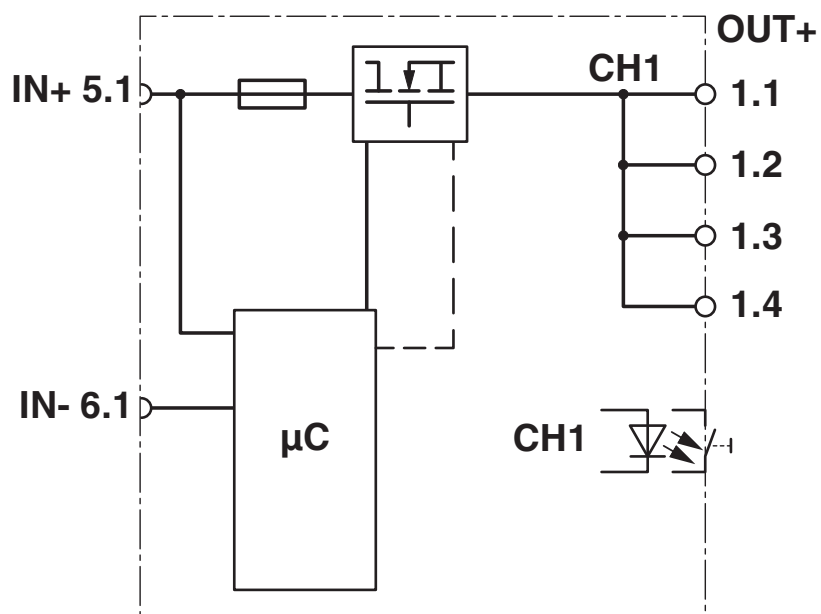
Schemat blokowy
