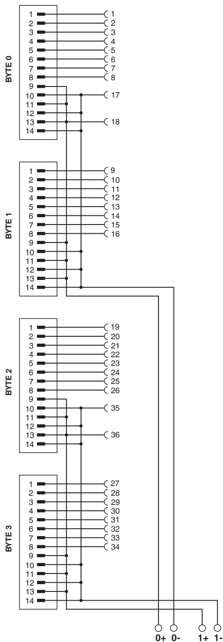
Schemat
