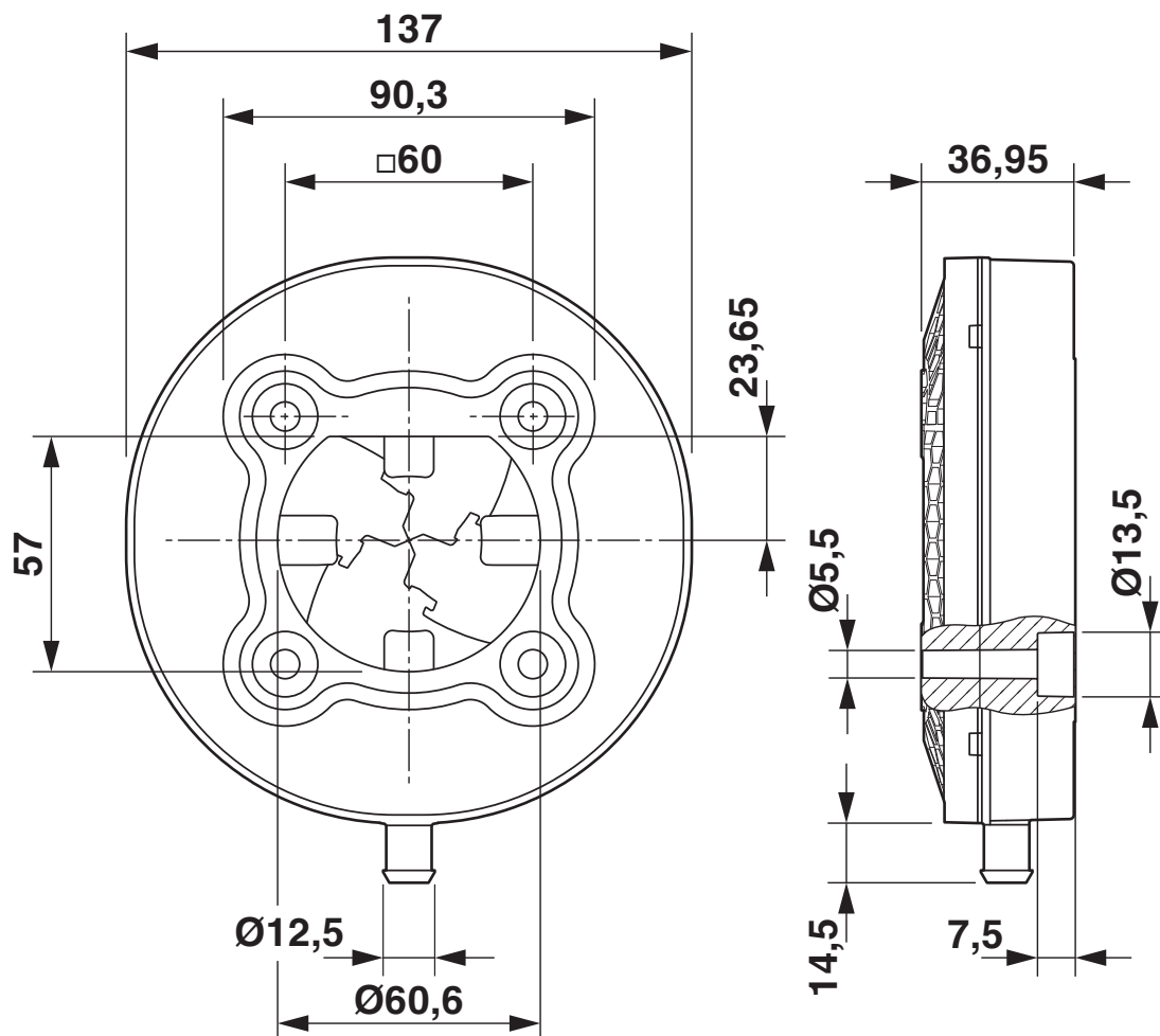
Rysunek wymiarowy
