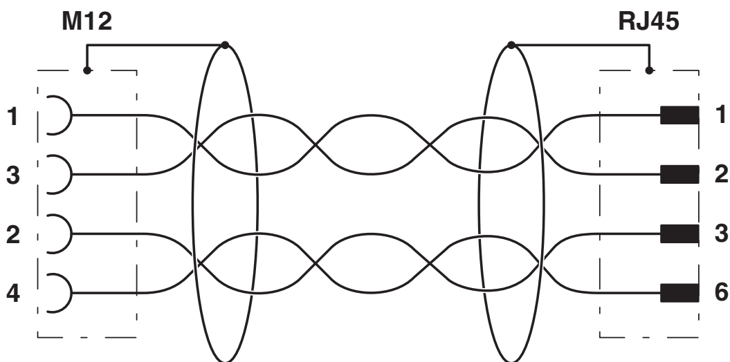
Przyporządkowanie styków gniazda M12 i wtyku RJ45
