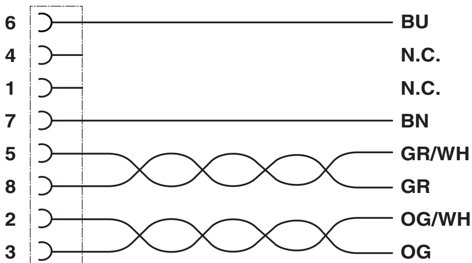
Przyporządkowanie styków gniazda M12
