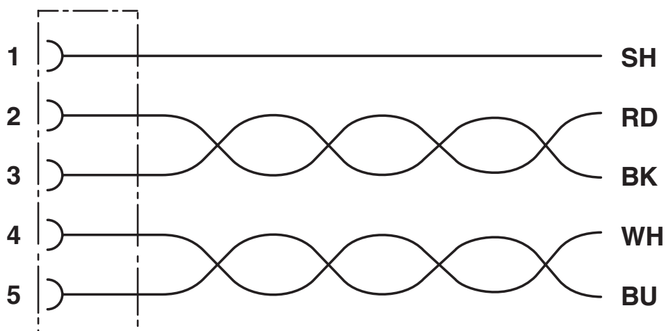
Przyporządkowanie styków gniazda M12
