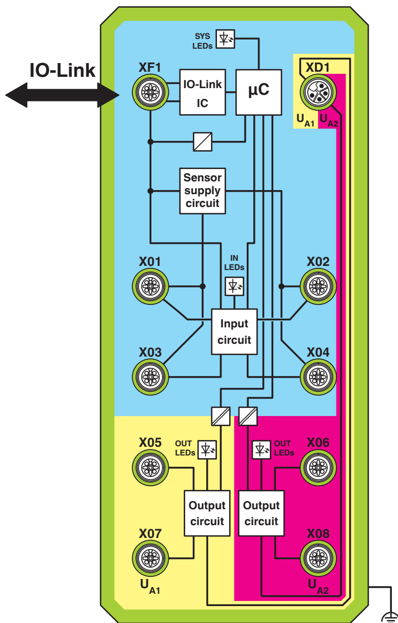
Schemat blokowy
