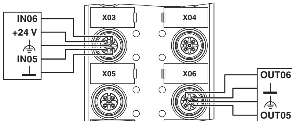
rysunek złączy
