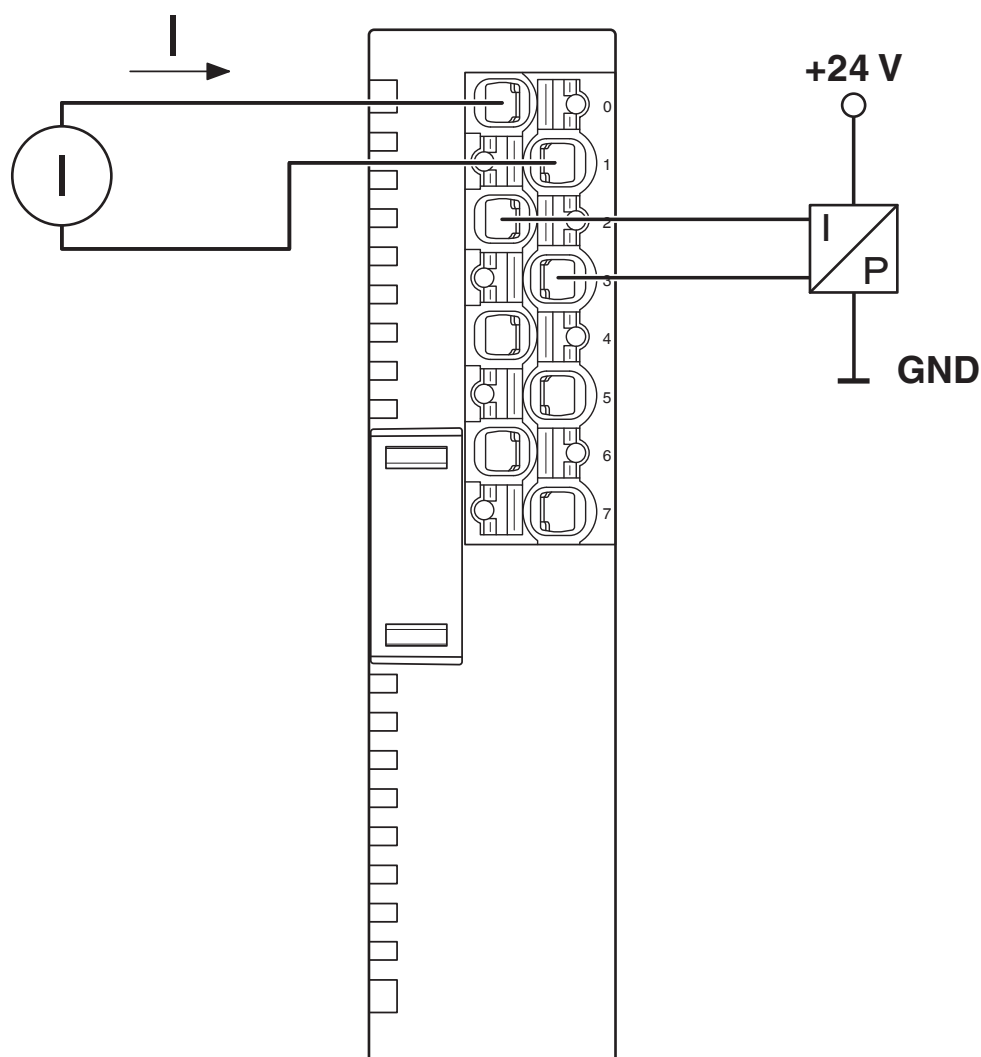
rysunek złączy
