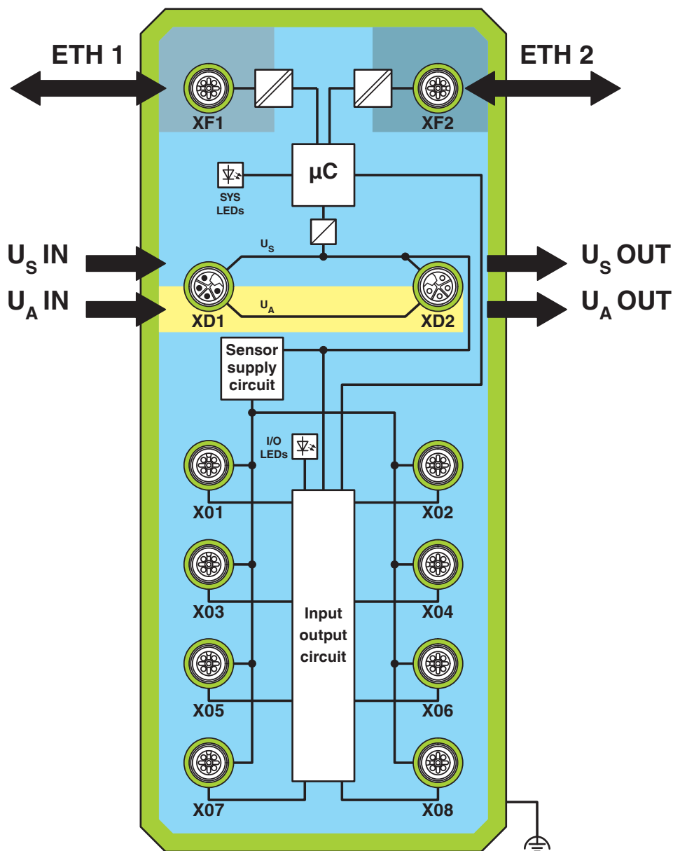
Schemat blokowy
