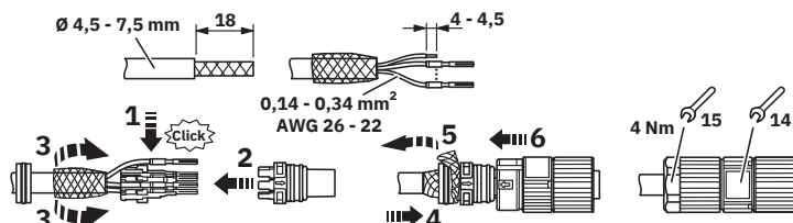
rysunek funkcyjny
