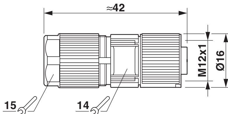
Wtyk z gniazdem M12 x 1, prosty, ekranowany
