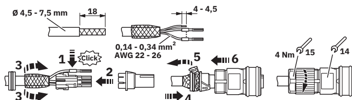
rysunek funkcyjny
