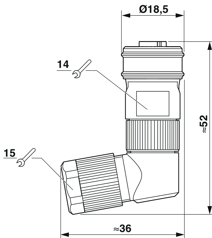
Rysunek wymiarowy
