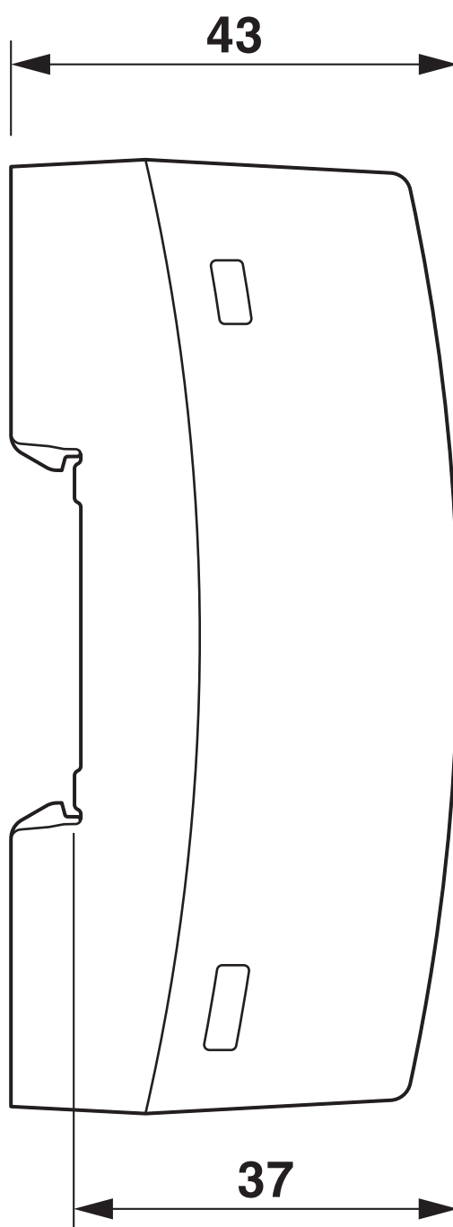
Rysunek wymiarowy
