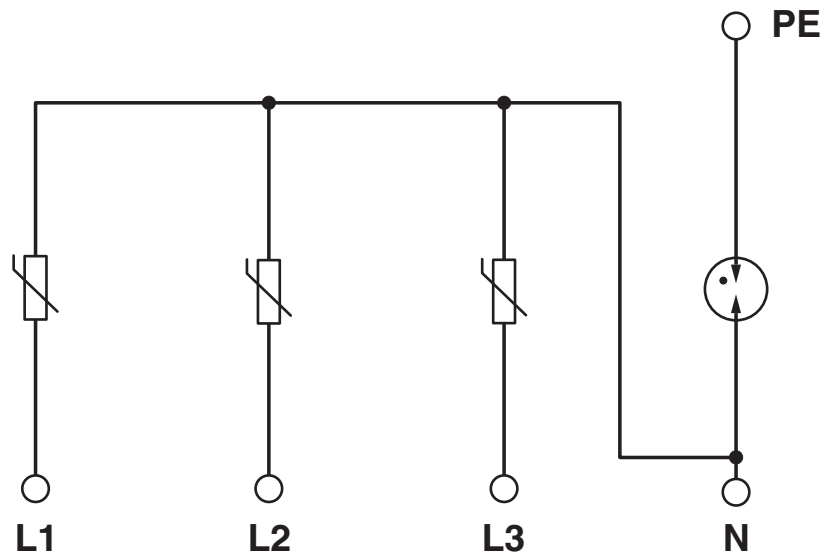
Schemat
