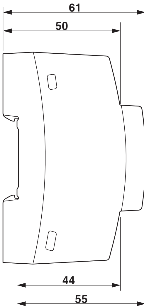
Rysunek wymiarowy
