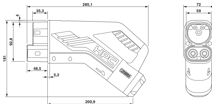
Rysunek wymiarowy
