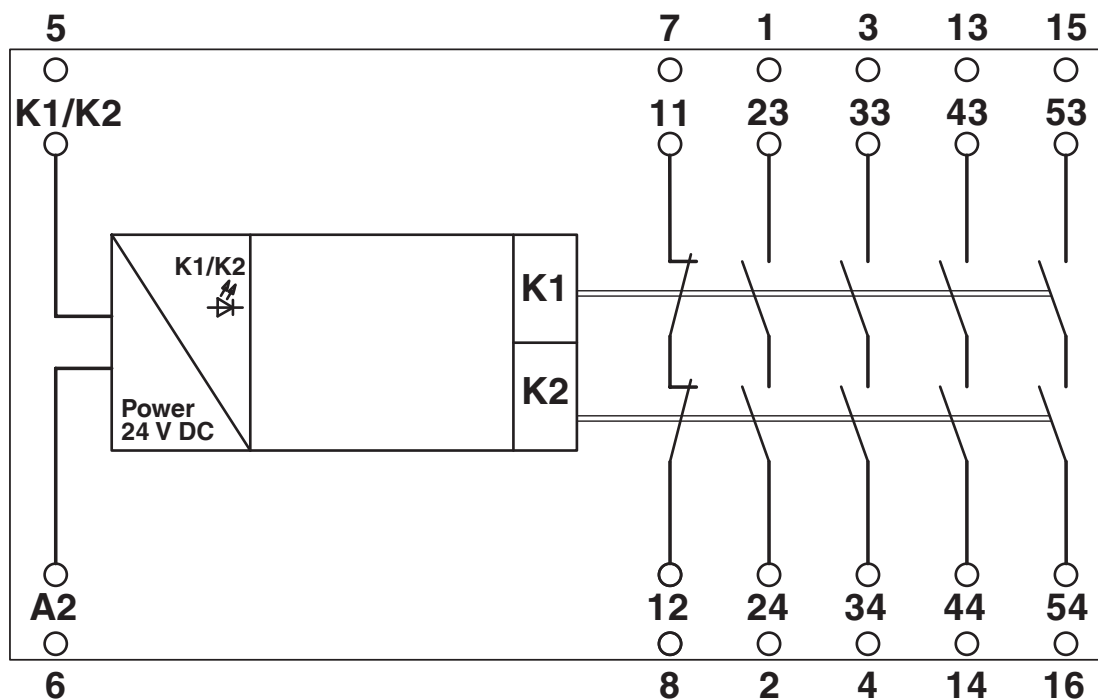
Schemat blokowy
