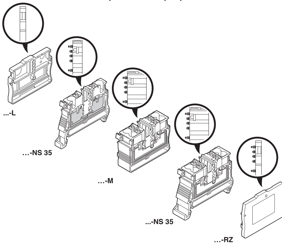
Rysunek schematyczny
