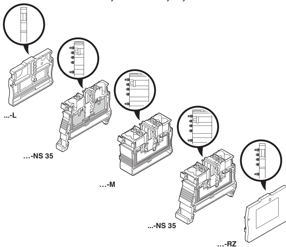
Rysunek schematyczny
