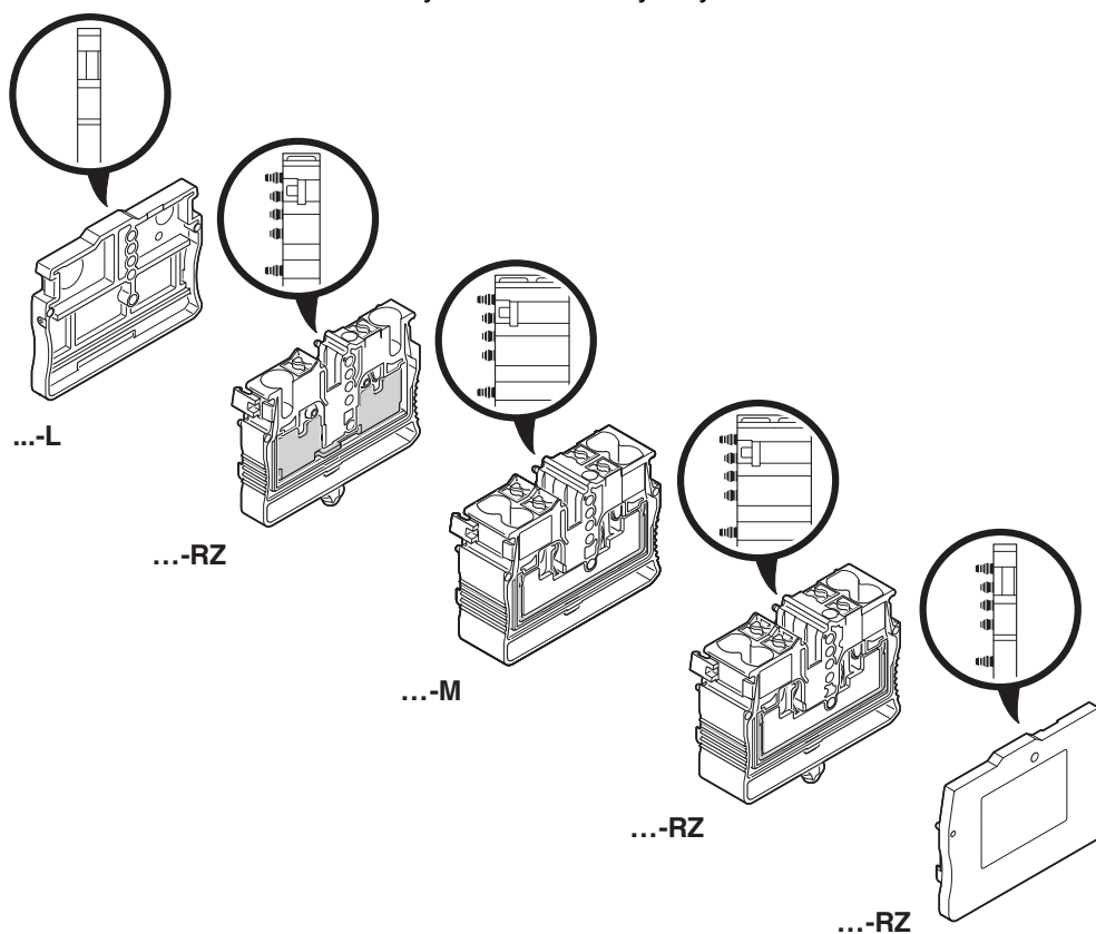
Rysunek schematyczny
