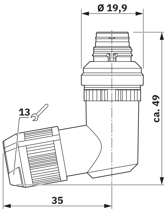
Rysunek wymiarowy
