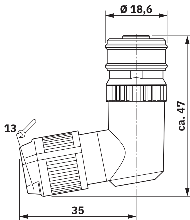
Rysunek wymiarowy
