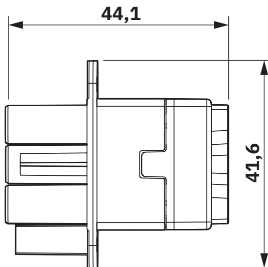
Rysunek wymiarowy
