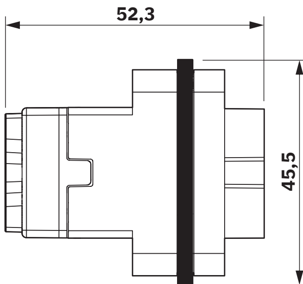
Rysunek wymiarowy
