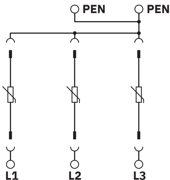
Schemat
