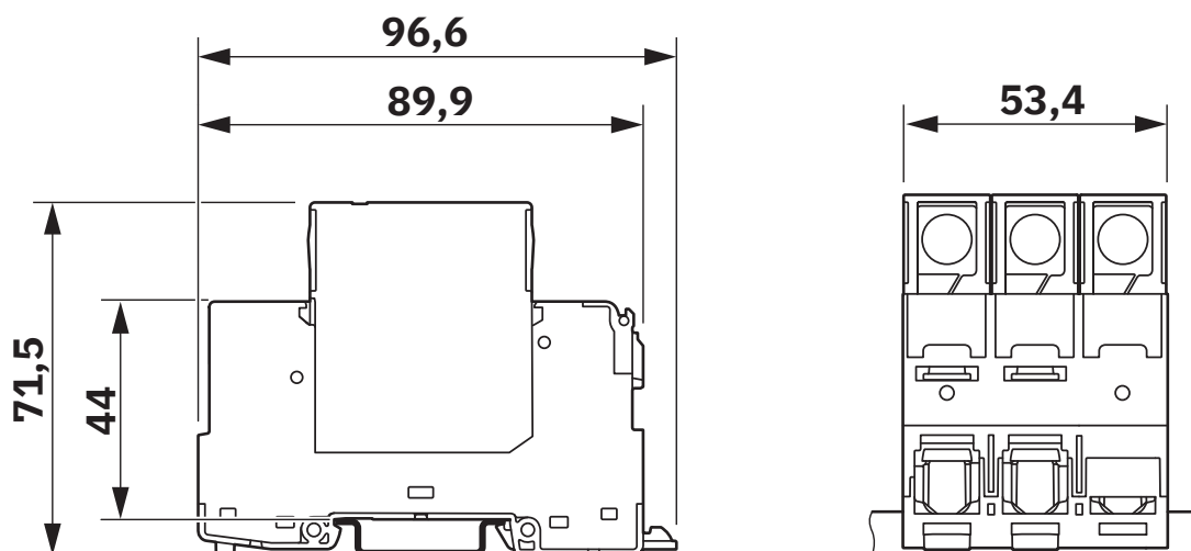
Rysunek wymiarowy
