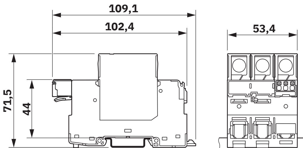
Rysunek wymiarowy
