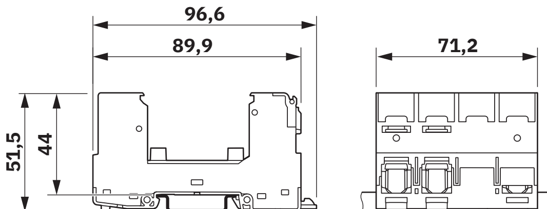
Rysunek wymiarowy
