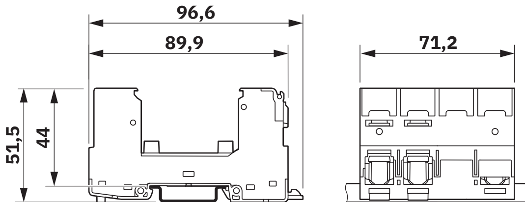
Rysunek wymiarowy
