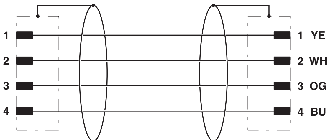
Przyporządkowanie styków wtyków M8
