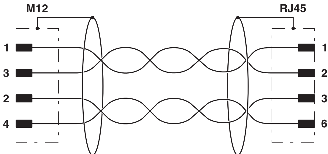
Przyporządkowanie styków wtyku M12 i RJ45
